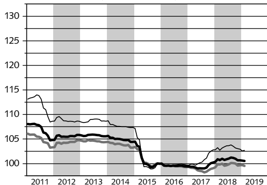
Indexverlauf (Kerninflation)
